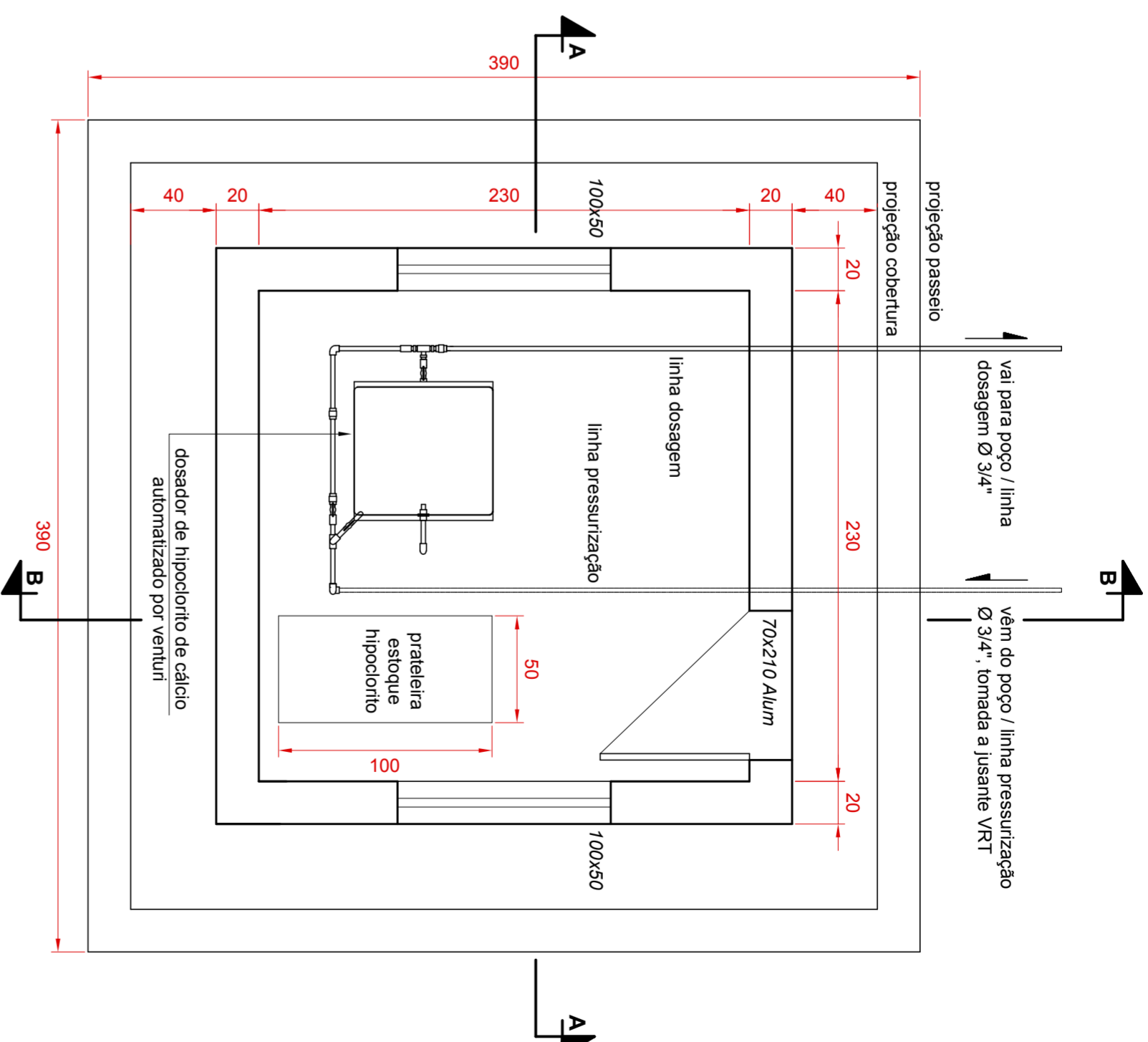
Casa Abrigo Dosador e Químicos - Planta Baixa Escala - 1 : 25
