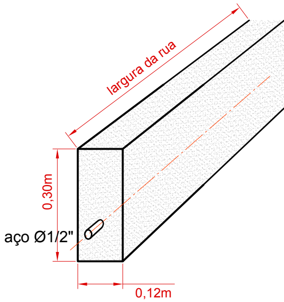
Viga de Contenção Sem Escala
