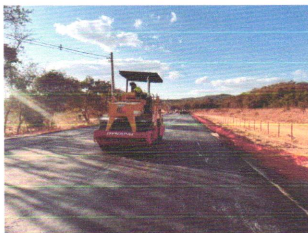
Foto 81 – Execução de pavimento com aplicação de concreto asfáltico.
