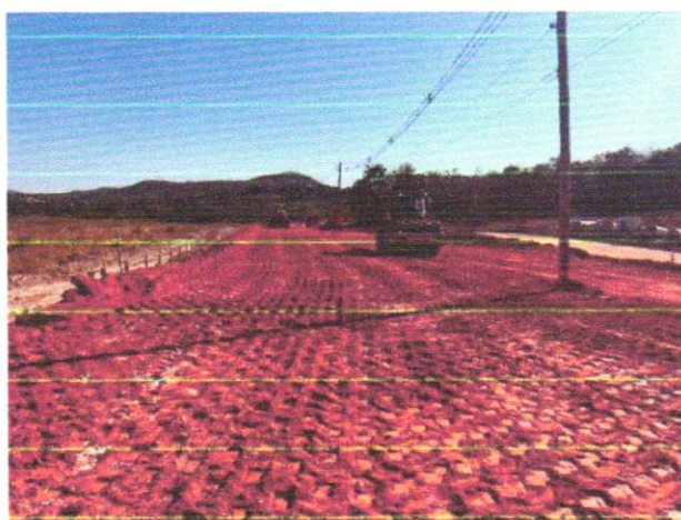
Foto 50 – Execução e compactação de aterro com solo predominantemente argiloso.
