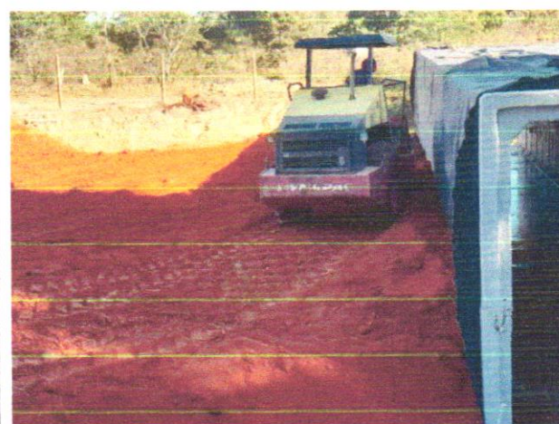
Foto 83 – Compactação de bueiro duplo celular de concreto 3,00x3,00 m.
