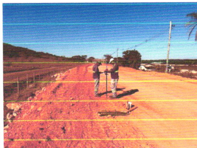
Foto 07 – Locação topográfica.
