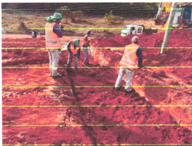
Foto 26 – Reaterro manual e compactação de vala.
