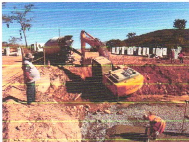
Foto 17 – Concretagem de Berço para bueiro duplo celular de concreto 3,00x3,00 m.
