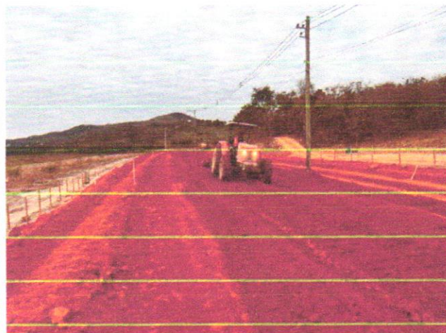
Foto 33 – Regularização e compactação de subleito.
