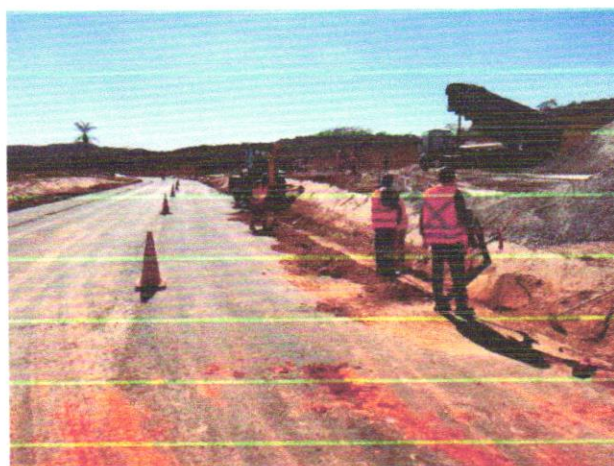
Foto 08 – Execução de Sarjeta triangular de concreto (STC-02).
