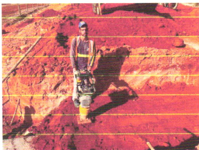
Foto 27- Reaterro manual e compactação de vala.
