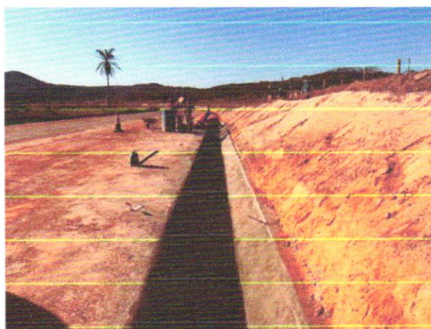
Foto 54 – Execução de Sarjeta triangular de concreto (STC-02).
