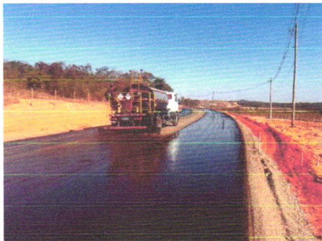
Foto 84 – Imprimação (Execução e Fornecimento do Material betuminoso).
