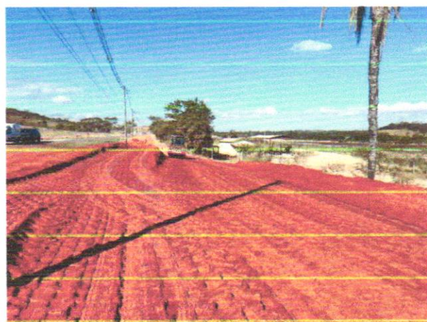
Foto 22 – Execução de Reforço de Subleito.
