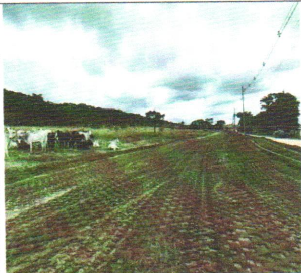
Foto 50 – Execução e compactação de aterro com solo predominantemente argiloso.
