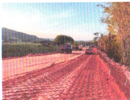
Foto 73 – Regularização e compactação de subleito. (Pista de caminhada)
