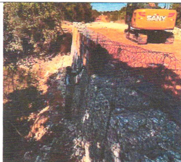
Foto 33 – Execução de arrimo em gabião tipo caixa.
