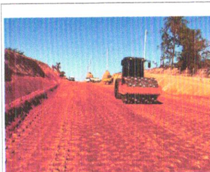
Foto 09 – Regularização e compactação de subleito.
