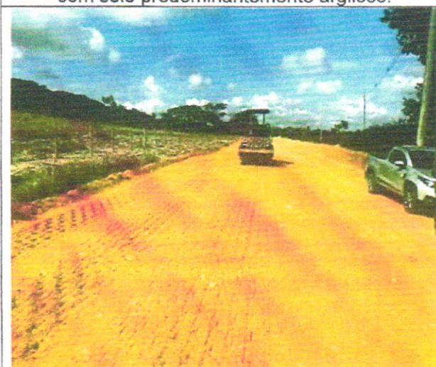
Foto 43 – Execução e compactação de aterro com solo predominantemente argiloso.
