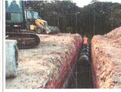
Foto 78 – Tubo de concreto DN 800 mm.
