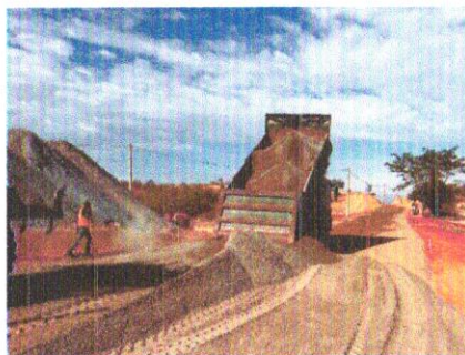
Foto 57 – Execução e compactação de base.
