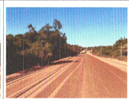
Foto 158 – Execução e compactação de base.
