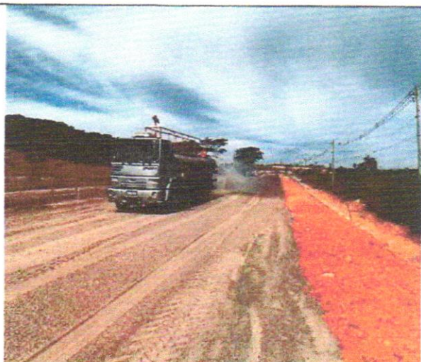
Foto 78 – Execução e compactação de base.
