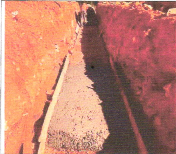
Foto 93 – Forma e concreto para berço tubular.
