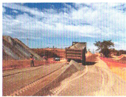
Foto 58 – Execução e compactação de base.
