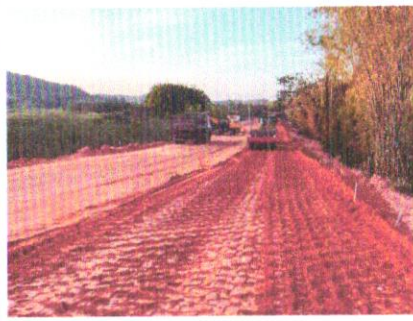
Foto 74 – Regularização e compactação de subleito. - (Pista de caminhada).
