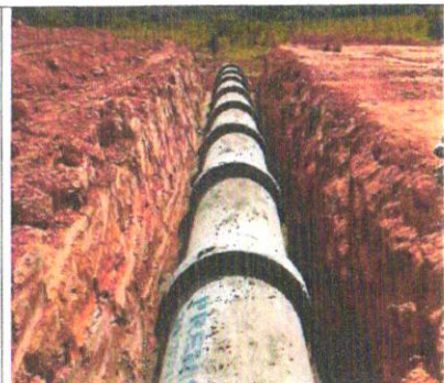
Foto 62 – Tubo de concreto DN 800 mm.
