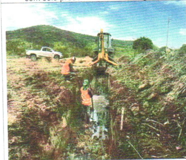
Foto 54 – Escavação mecanizada de vala.
