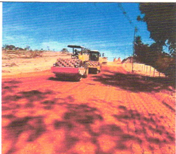
Foto 46 – Execução e compactação de aterro com solo predominantemente argiloso.
