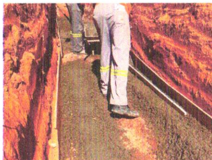
Foto 67 – Forma e concreto para berço tubular.
