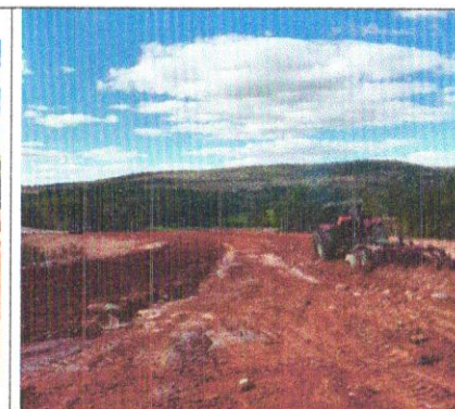
Foto 118 – Execução e compactação de subleito.
