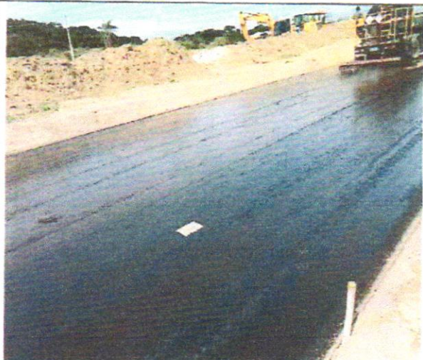
Foto 86 – Imprimação asfáltica.
