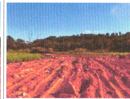
Foto 62 – Execução e compactação de aterro.
