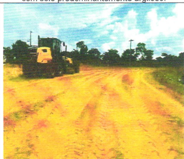
Foto 44 – Execução e compactação de aterro com solo predominantemente argiloso.
