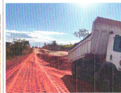
Foto 56 – Execução de camada final de aterro..
