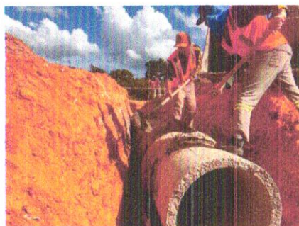
Foto 89 – Execução de contra-berço.
