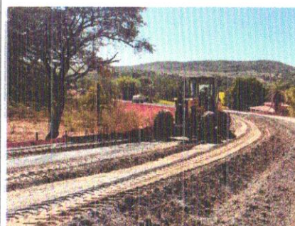
Foto 127 – Regularização e compactação de subleito.
