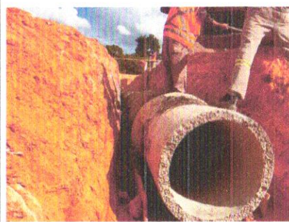
Foto 90 – Execução de contra-berço.
