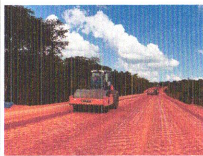
Foto 92 – Regularização e compactação de subleito.
