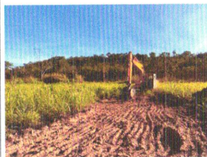
Foto 34 – Desmatamento, destocamento, limpeza de área.
