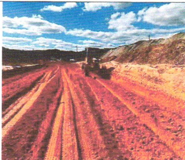
Foto 58 – Regularização e compactação de subleito.
