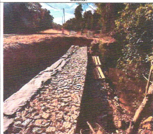
Foto 31 – Execução de arrimo em gabião tipo caixa.
