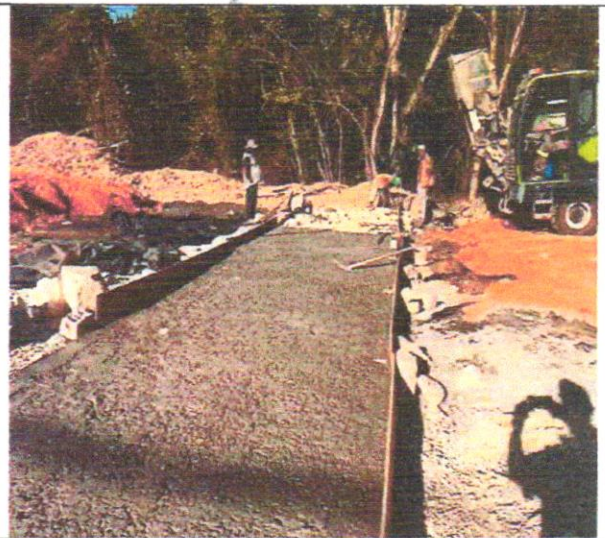
Foto 94 – Forma e concreto para berço tubular.
