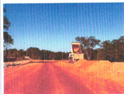
Foto 11 – Execução e compactação de aterro com solo predominantemente argiloso.
