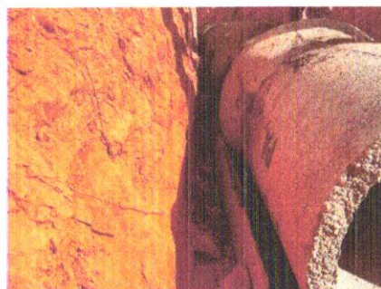
Foto 91 – Execução de contra-berço.
