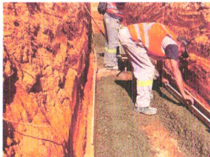
Foto 68 – Forma e concreto para berço tubular.
