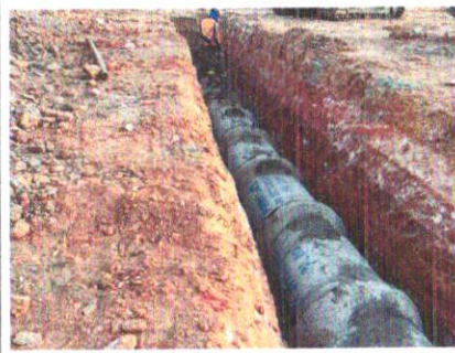
Foto 76 – Tubo de concreto DN 800 mm.
