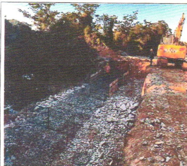
Foto 29 – Execução de arrimo em gabião tipo caixa.
