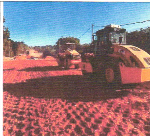
Foto 49 – Execução e compactação de aterro com solo predominantemente argiloso.
