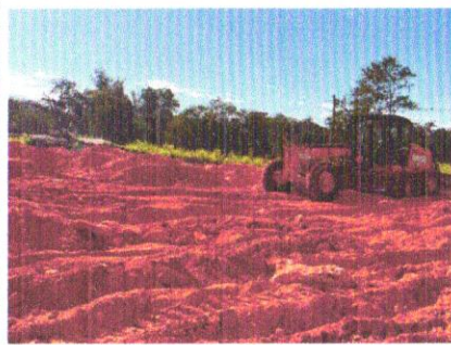
Foto 60 – Execução e compactação de aterro.
