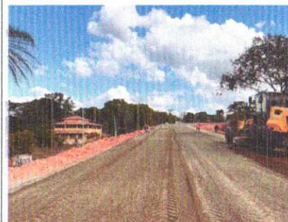
Foto 143 - Execução e compactação base.
