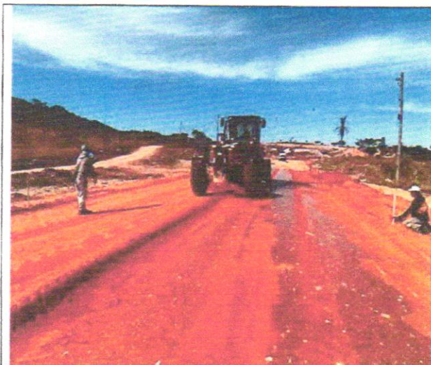
Foto 65 – Regularização e compactação de subleito.
