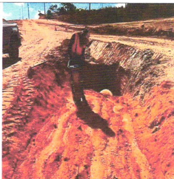
Foto 102 – Reaterro manual e compactação de vala.
