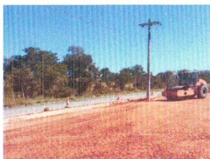
Foto 123 – Execução e compactação de subleito.
