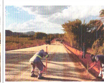
Foto 150 – Confêrencia e nivelamento feito pela fiscalização
