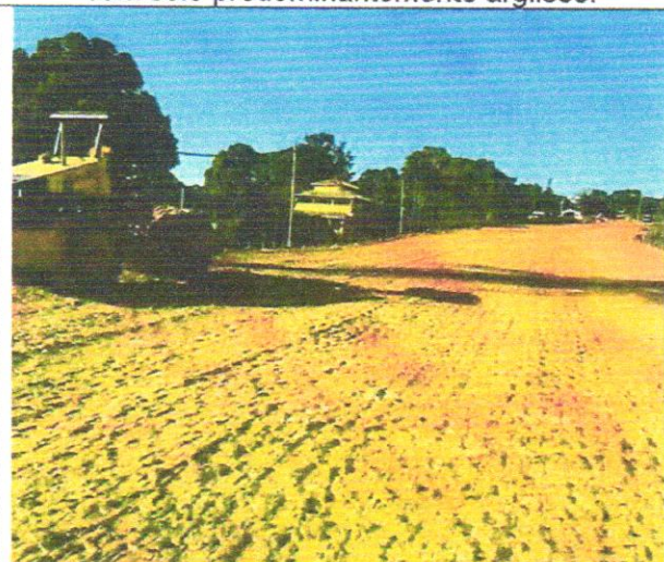
Foto 47 – Execução e compactação de aterro com solo predominantemente argiloso.
