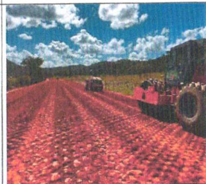
Foto 48 – Execução e compactação de aterro com solo predominantemente argiloso. Estaca 90 a 100.
