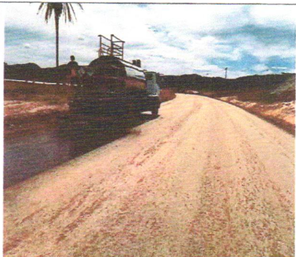
Foto 82 – Imprimação asfáltica.
