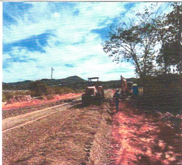
Foto 68 – Execução e compactação de sub-base.
