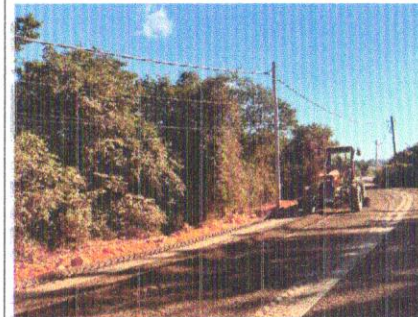
Foto 159 – Execução e compactação de base.
