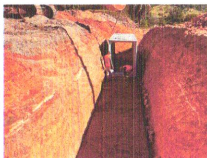
Foto 121 – Execução de Passa gado.
