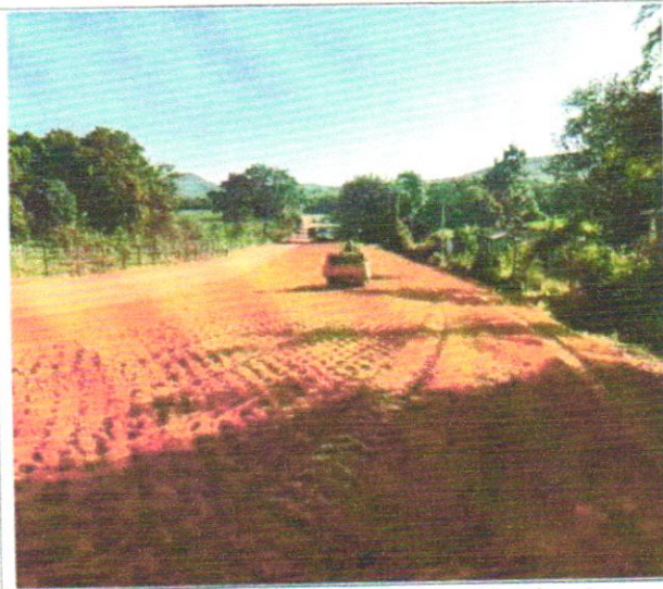
Foto 53 – Execução e compactação de aterro com solo predominantemente argiloso.
