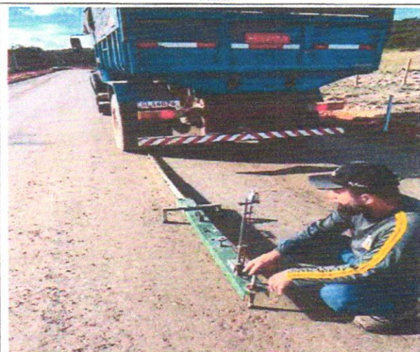
Foto 103 – Ensaios laboratoriais de viga benkelman, liberação de base em BGS.
