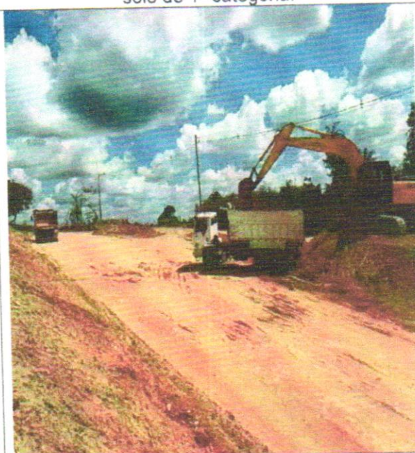
Foto 44 – Escavação vertical a céu aberto em solo de 1ª categoria.
