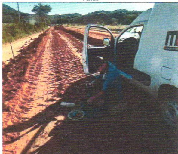
Foto 104 – Liberação camada de aterro escalonamento
