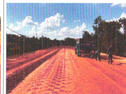
Foto 96 – Liberação camada de subleito.
