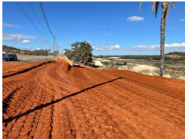
Foto 22 – Execução de Reforço de Subleito.
