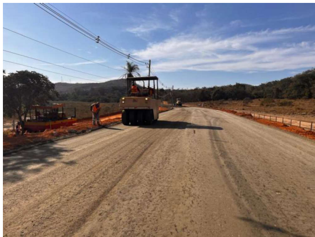
Foto 61 – Execução e compactação de base
