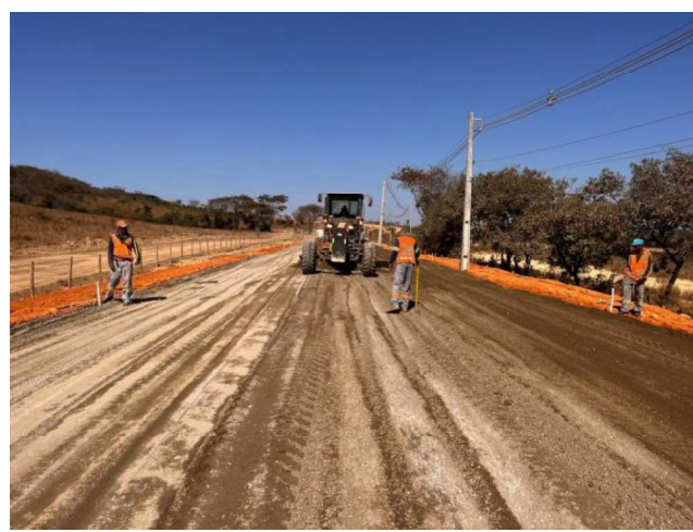
Foto 58 – Execução e compactação de base.
