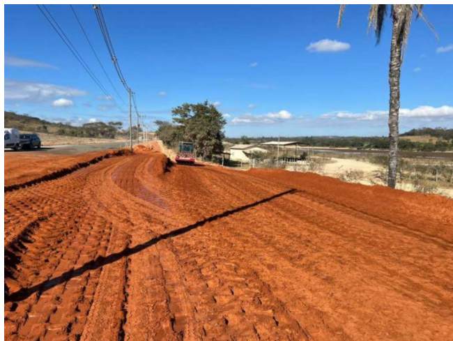
Foto 23 – Execução de Reforço de Subleito.
