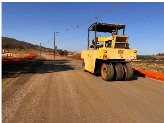
Foto 55 – Execução e compactação de sub-base.
