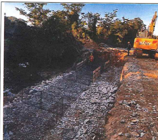
Foto 29 – Execução de arrimo em gabião tipo caixa.
