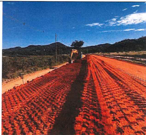
Foto 50 – Escalonamento e levantamento topográfico.
