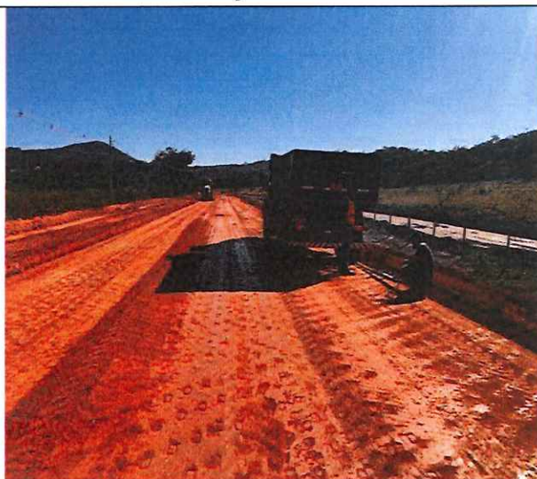
Foto 108 – Liberação camada de subleito
