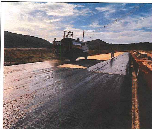
Foto 85 – Imprimação asfáltica.
