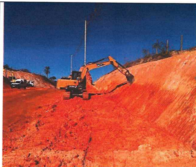
Foto 57 – Execução de rampa 1x1.
