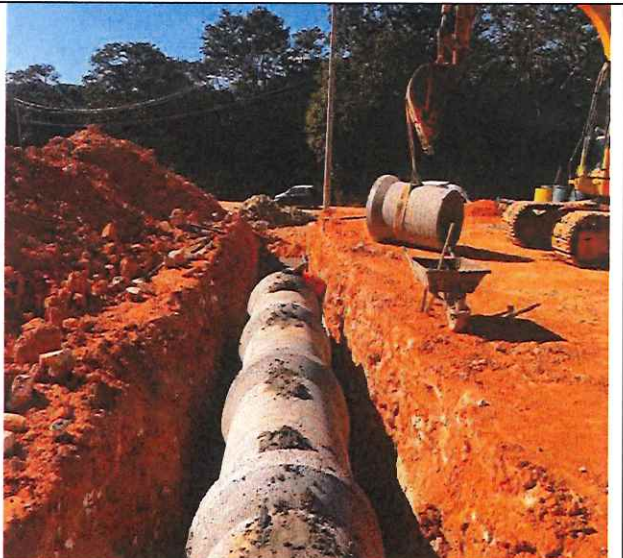
Foto 96 – Tubo de concreto DN 800 mm.
