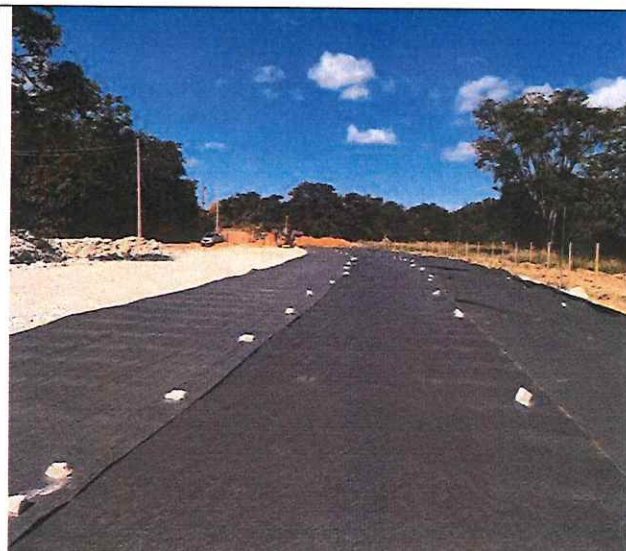
Foto 89 – Aplicação de manta bidim.
