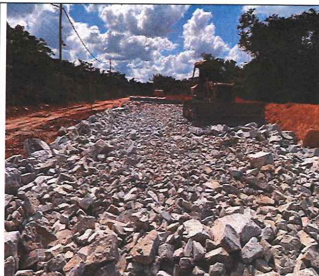
Foto 25 – Enrocamento com pedra de mão.
