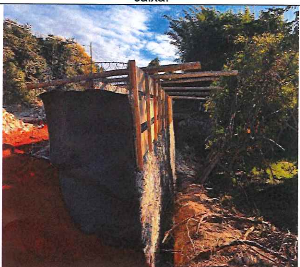
Foto 32 – Execução de arrimo em gabião tipo caixa.
