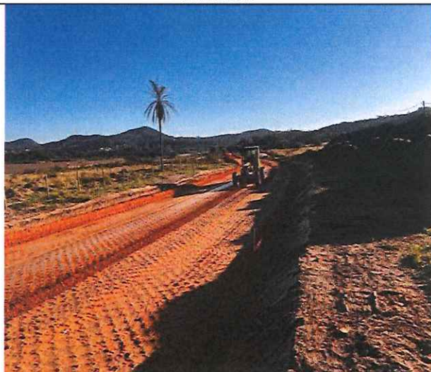
Foto 64 – Regularização e compactação de subleito.
