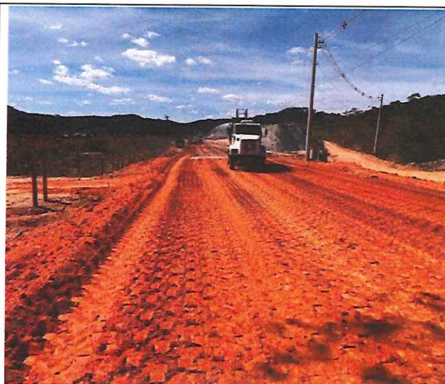
Foto 45 – Execução e compactação de aterro com solo predominantemente argiloso.
