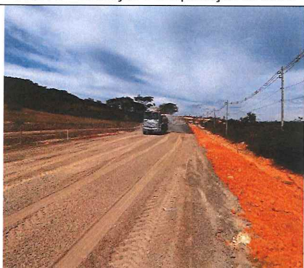
Foto 80 – Execução e compactação de base.
