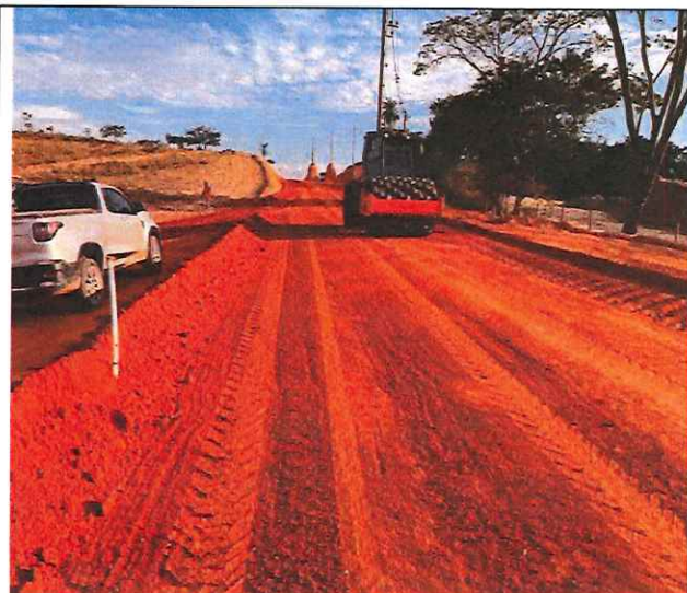
Foto 61 – Regularização e compactação de subleito.
