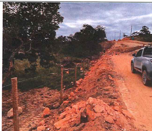
Foto 21 – Remoção de cercas e mourões.
