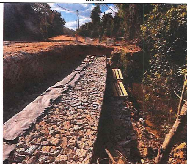
Foto 31 – Execução de arrimo em gabião tipo caixa.
