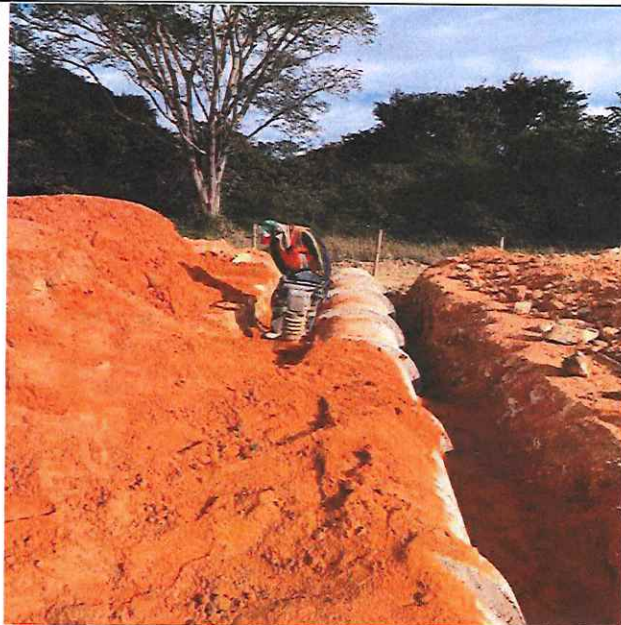
Foto 101 – Reaterro manual e compactação de vala.
