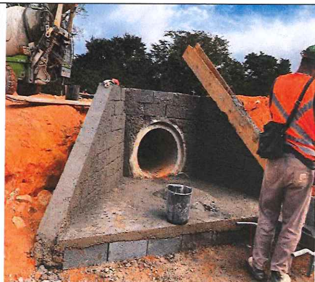
Foto 114 – Execução de ala.
