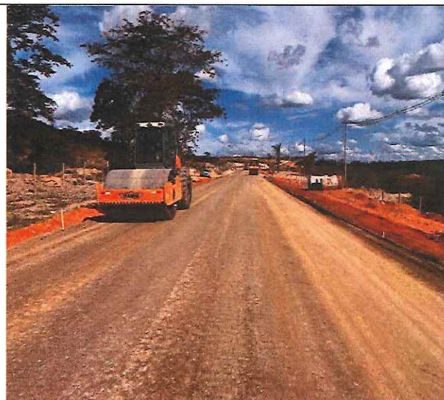
Foto 75 – Execução e compactação de sub-base.
