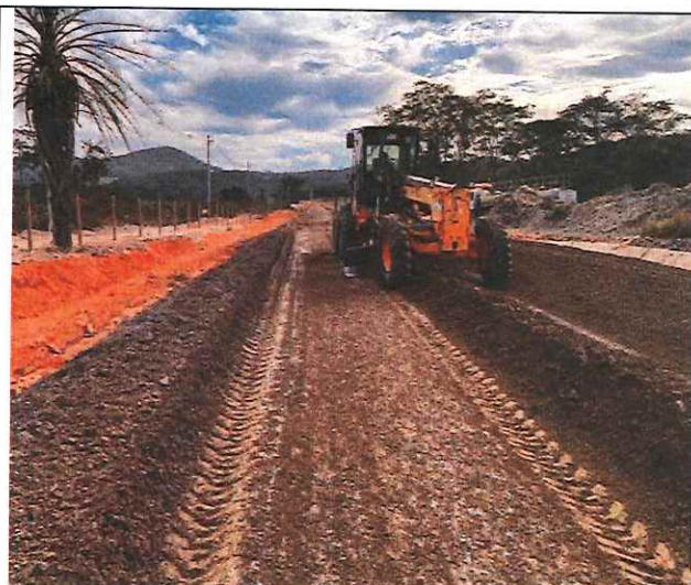
Foto 77 – Execução e compactação de base.
