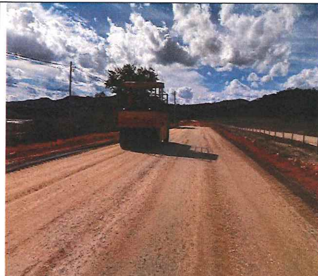
Foto 73 – Execução e compactação de sub-base.
