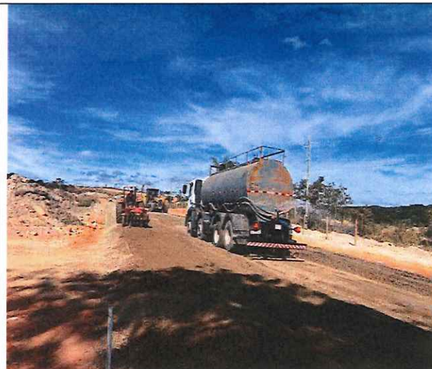
Foto 70 – Execução e compactação de sub-base.
