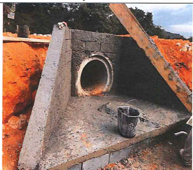
Foto 112 – Execução de ala.
