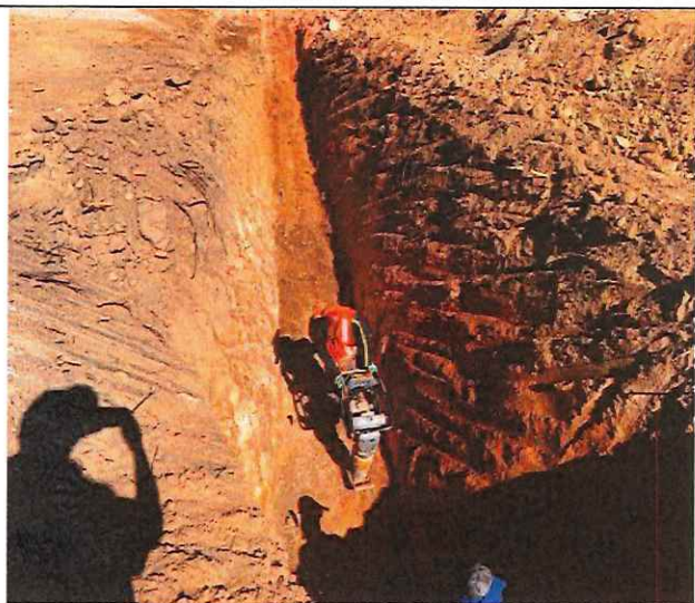
Foto 92 – Compactação de fundo de vala.
