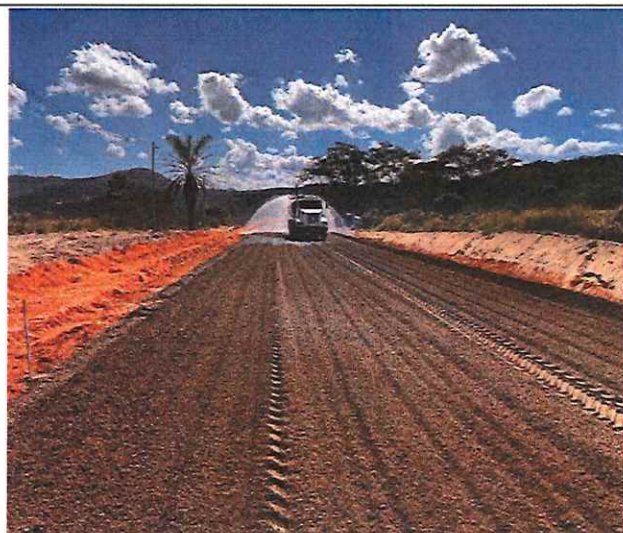
Foto 69 – Execução e compactação de sub-base.
