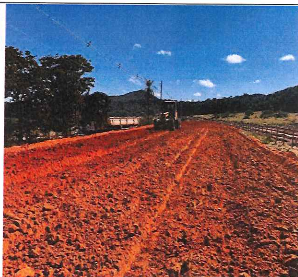
Foto 54 – Execução de camada final de aterro.
