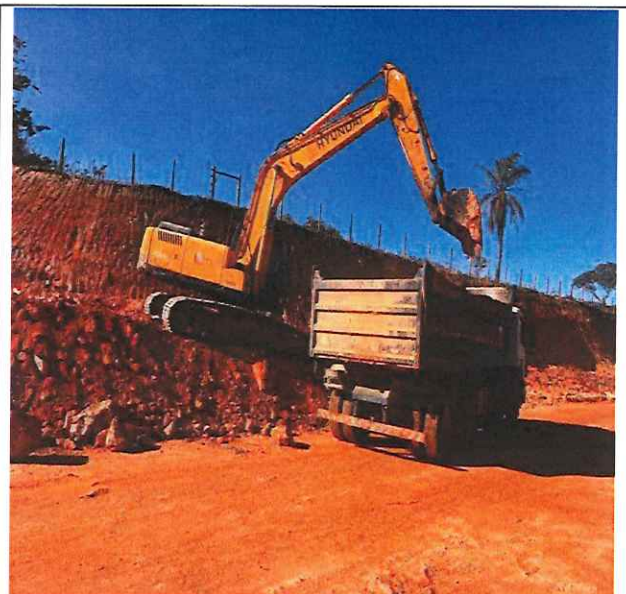
Foto 42 – Escavação, carga e transporte de material de 2ª categoria.
