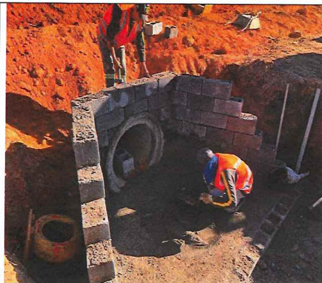
Foto 113 – Execução de ala.
