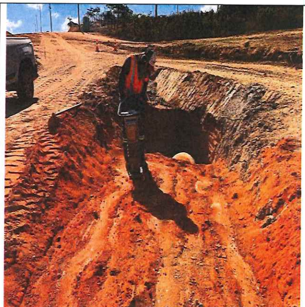
Foto 102 – Reaterro manual e compactação de vala.
