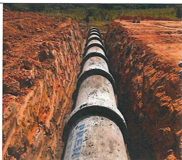
Foto 62 – Tubo de concreto DN 800 mm.
