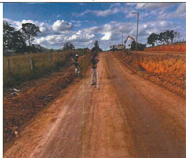
Foto 07 – Locação topográfica.
