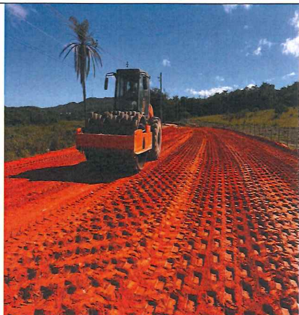
Foto 50 – Execução e compactação de aterro com solo predominantemente argiloso. Estaca 83 a 92.
