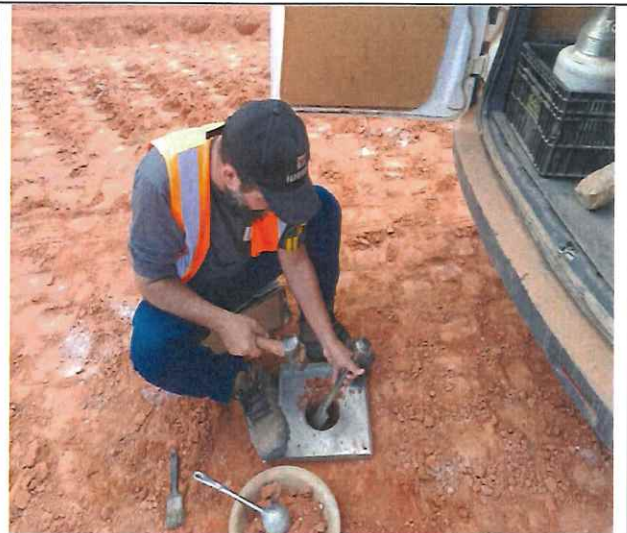
Foto 66 – Ensaios laboratoriais.
