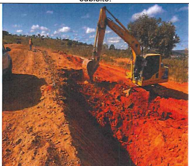
Foto 44 – Execução de rampa 1x1. Estaca 13 até 25 LE – Acesso Pedreira.
