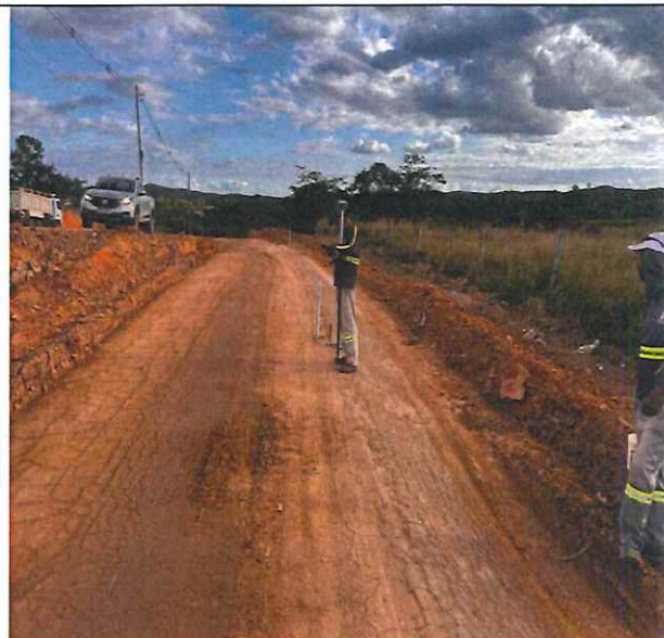
Foto 06 – Locação topográfica.
