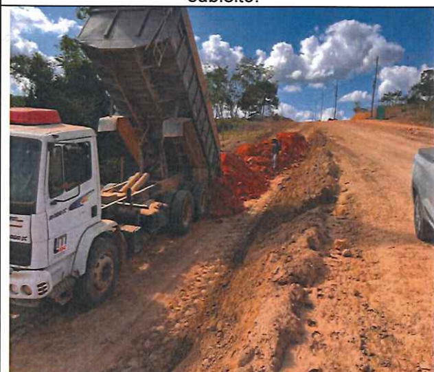
Foto 43 – Execução de corpo de aterro.
