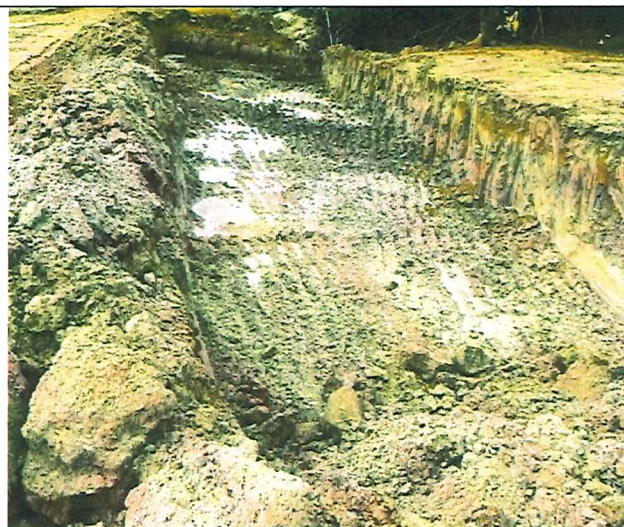
Foto 33 – Escavação mecânica em solo mole.
