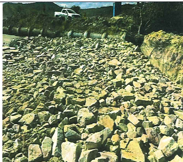
Foto 26 – Enrocamento com pedra de mão.
