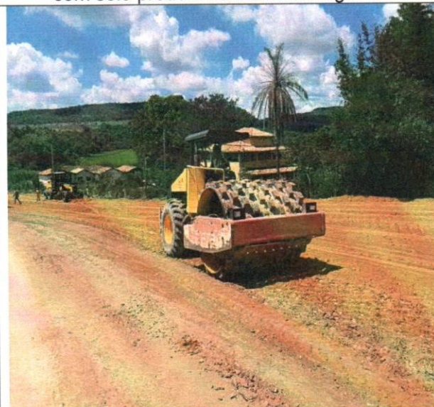
Foto 51 – Execução e compactação de aterro com solo predominantemente argiloso.
