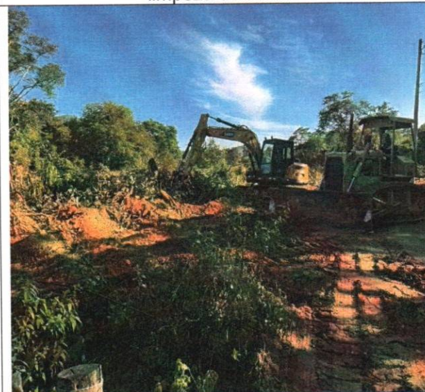
Foto 15 – Desmatamento, destocamento, limpeza de área.
