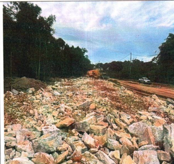
Foto 40 – Enrocamento com pedra de mão.
