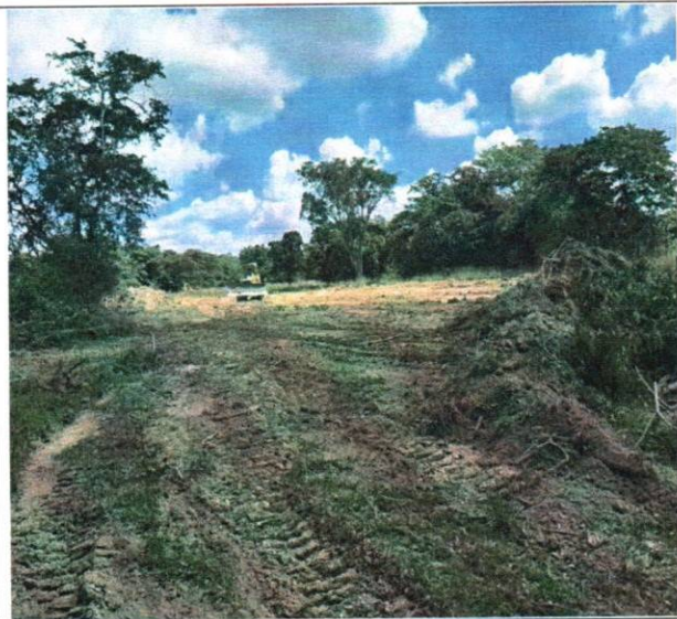
Foto 13 – Desmatamento, destocamento, limpeza de área.
