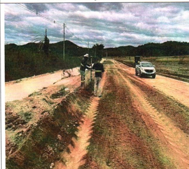
Foto 07 – Locação topográfica.
