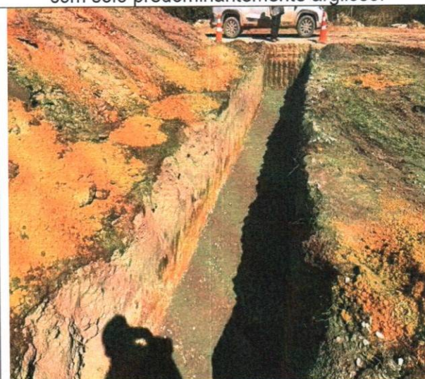
Foto 55 – Escavação mecanizada de vala e concreto para berço.
