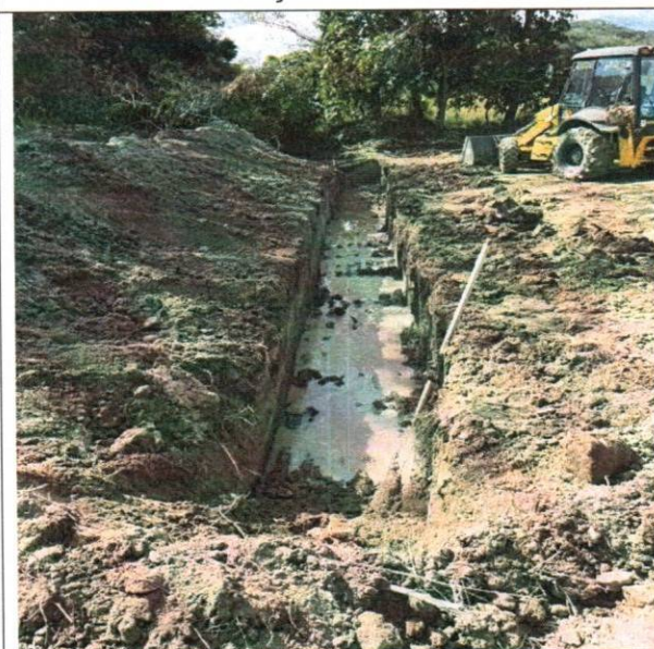
Foto 36 – Escavação mecânica em solo mole.
