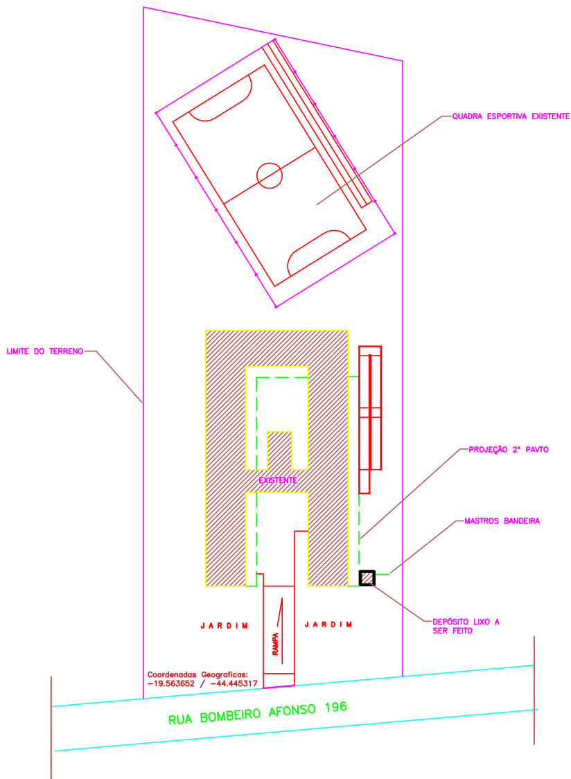
PLANTA DE SITUAÇÃO ESCALA 1/400
